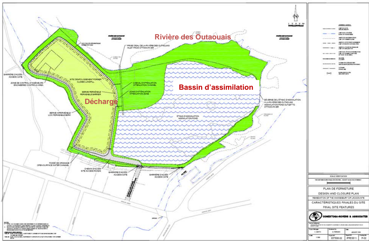
Figure 1 : Plan de réhabilitation à l'échelle réelle de l'étang de rétention de Hawkesbury
